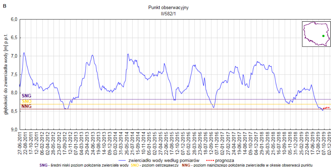
Rys. 15. Prognoza dotycząca stanu wód o zwierciadle swobodnym (gruntowych) na okres 01.11.2019 – 30.11.2019 r. – stacja hydrogeologiczna nr II/582/1 w miejscowości Bronowice (woj. lubelskie). A - prognoza przy założeniu scenariusza A; B - prognoza przy założeniu scenariusza B
