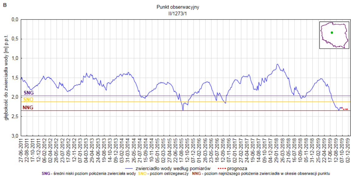
Rys. 8. Prognoza dotycząca stanu wód o zwierciadle swobodnym (gruntowych) na okres 01.11.2019 - 30.11.2019 r. – stacja hydrogeologiczna nr II/1273/1 w miejscowości Łuszczewo (woj. wielkopolskie). A - prognoza przy założeniu scenariusza A; B - prognoza przy założeniu scenariusza B
