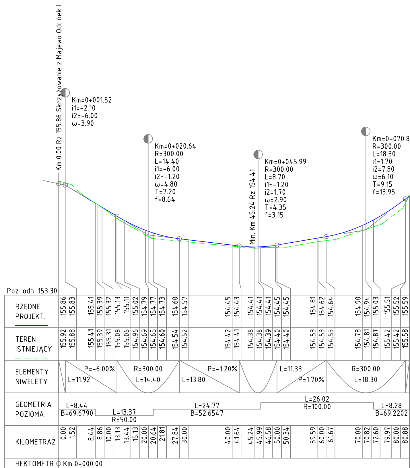
PROFIL PODŁUŻNY Majewo Odcinek II Km 0.000 to Km 80.881 Skala: POZIOMA 1:500 PIONOWA 1:50 Majewo Odcinek II
