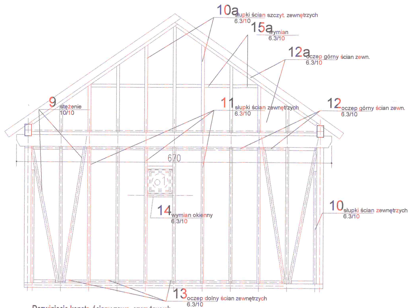
Rozwinięcie konstr. ściany zewn. szczytowych
