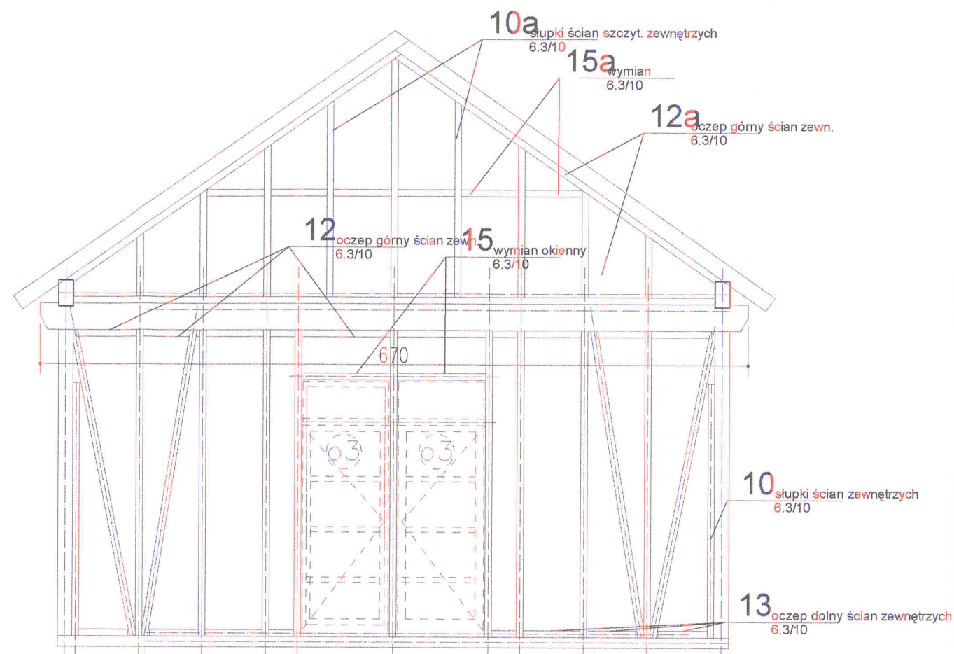
Rozwinięcie konstr. ściany zewn. szczytowych
