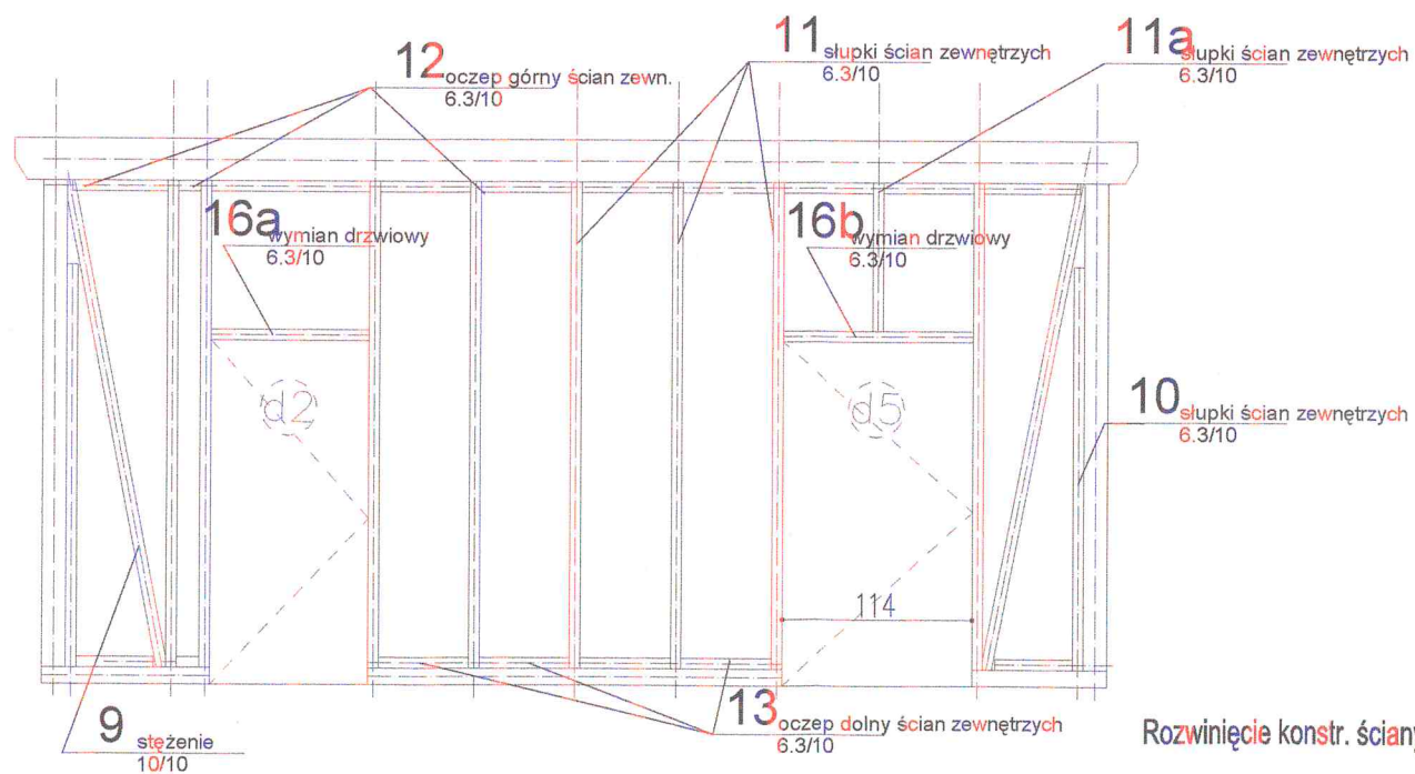
Rozwinięcie konstr. ściany zewn. szczytowych
